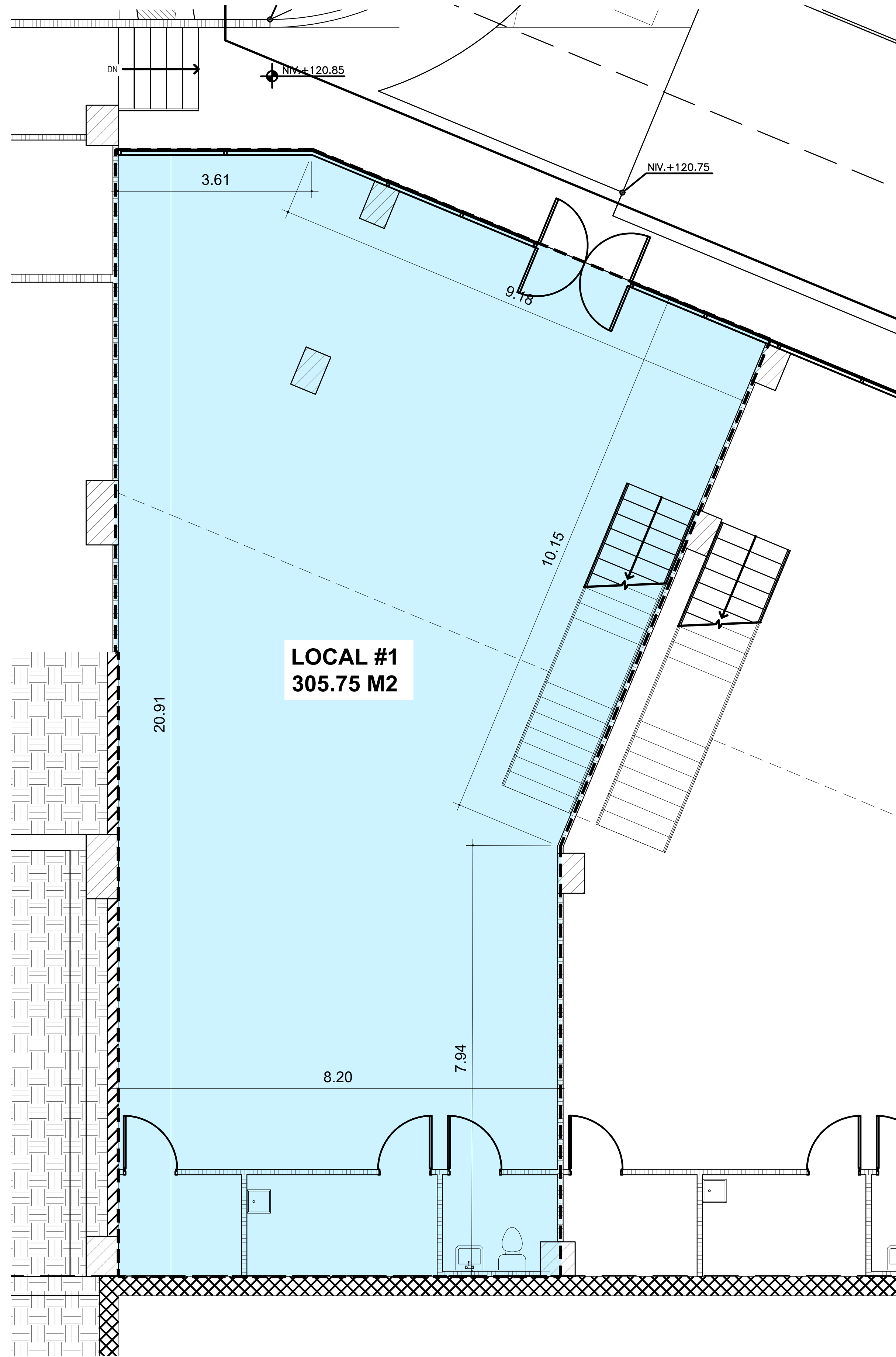
PLANTA ARQUITECTONICA ESC:1/50 LOCAL #1 NIVEL -050
